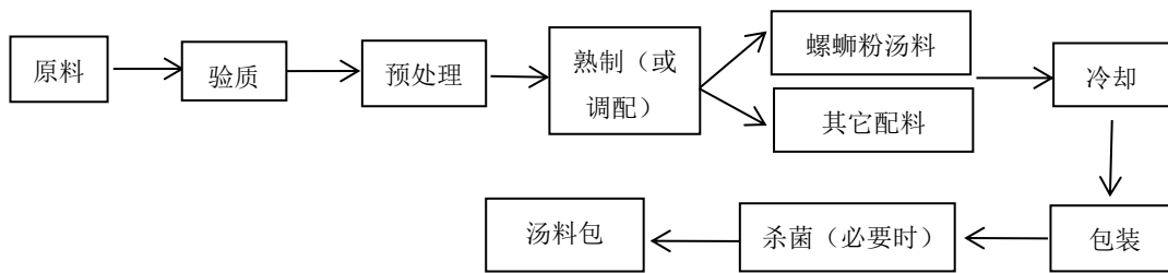
图 1 汤料包生产工艺流程图
