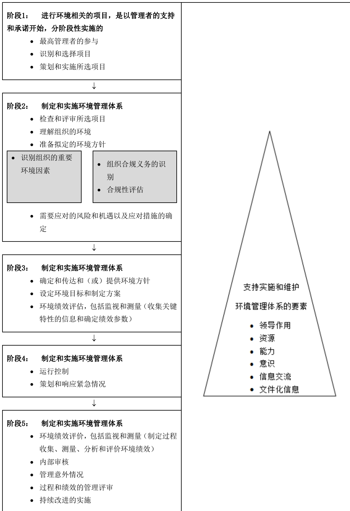
图 B.1——以五个阶段实施的示例
