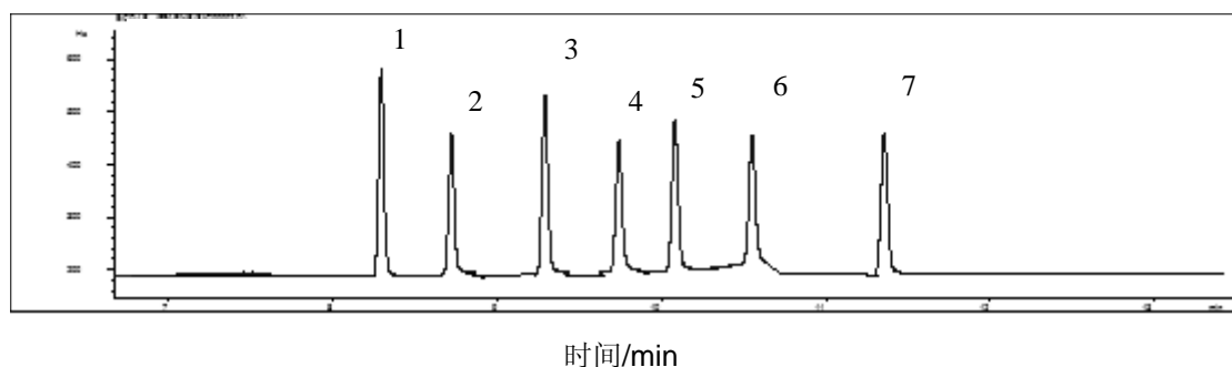
图 1. 硝基苯类化合物在 DB-FFAP 柱上的标准色谱图
