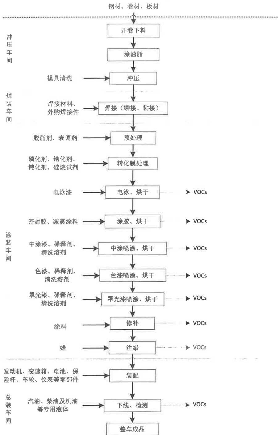
图 37-1 汽车整车制造生产流程图
