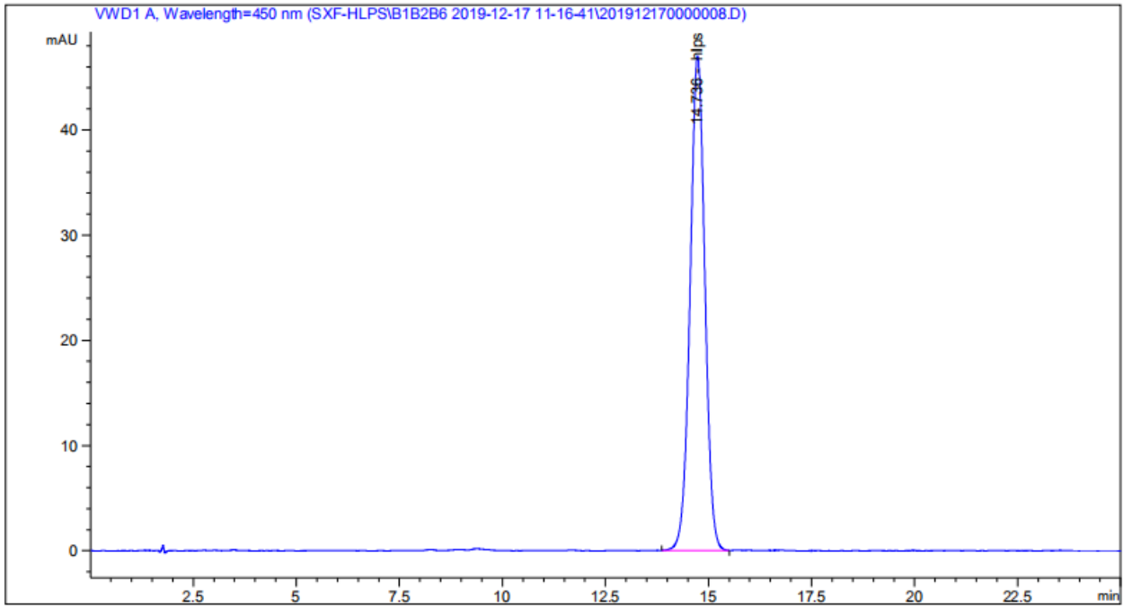
图 B.1 β-胡萝卜素标准溶液 (6.657 μg/mL) 的高效液相色谱图
